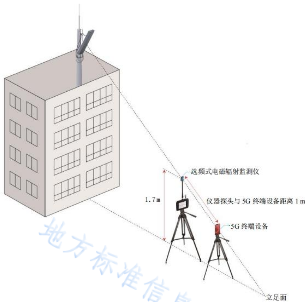
图 C.1 天线可视范围内的位置关系
